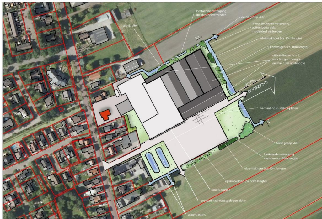
ERFINRICHTINGSSCHETS
